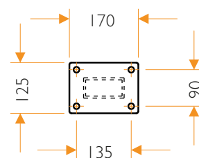
Baseplate
